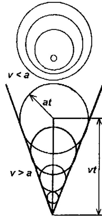
Рис. 3.1.5-2. Схема распространения звуковых волн от движущегося объекта в воздушной среде ( v – скорость движения объекта, a – скорость звука в воздухе, t – время)
