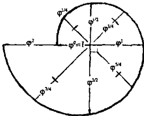
Рис. 2.1-2. Раскручивание спирали нашей Галактики по степеням коэффициента Золотого Сечения \Phi , кратным 1/4
