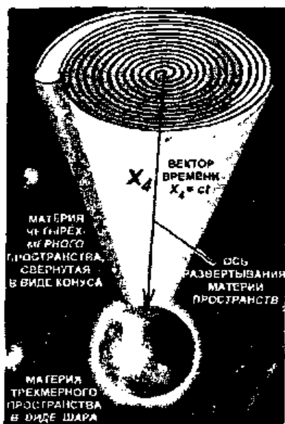
Рис. 3.1.3-4. Схема развёртывания материи трёхмерного пространства в материю четырёхмерного пространства на примере матрицы Земного шара
