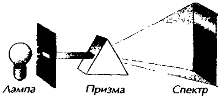
Рис. 3.6-1. Разложение белого света кристаллом призмы на спектр цветов
