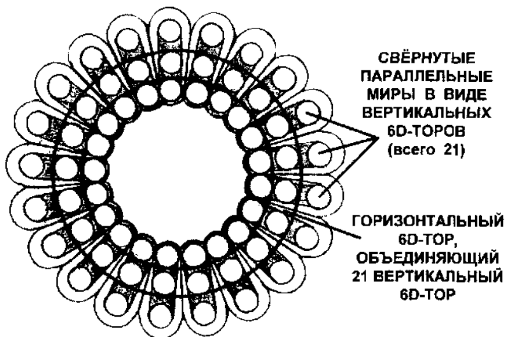
Рис. 3.1.3-7 Б. Схема строения семимерного пространства. Горизонтальный разрез 7D-тори
