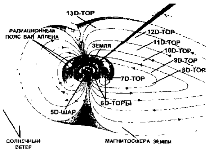
Рис. 3.1.4-3. Схема строения магнитосферы Земли с аналогами форм многомерных пространств
